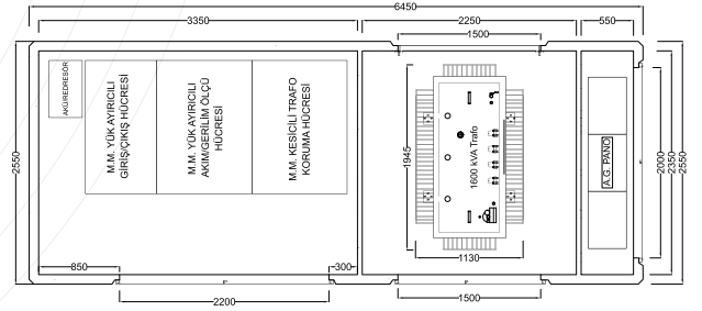
MBK 6450/1600
