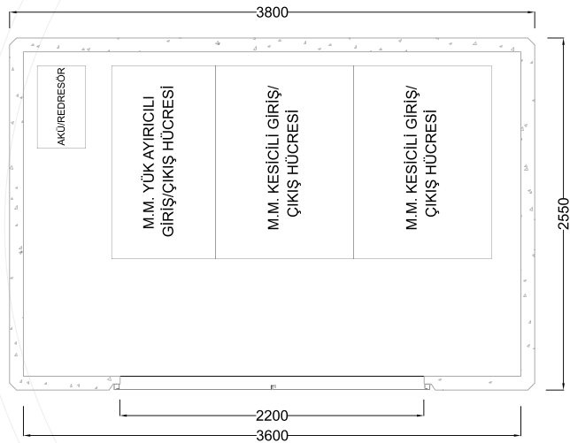
MBK 3800/DM
