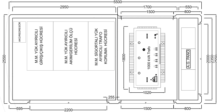
MBK 5500/1000
