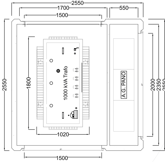
MBK 2500/1000
